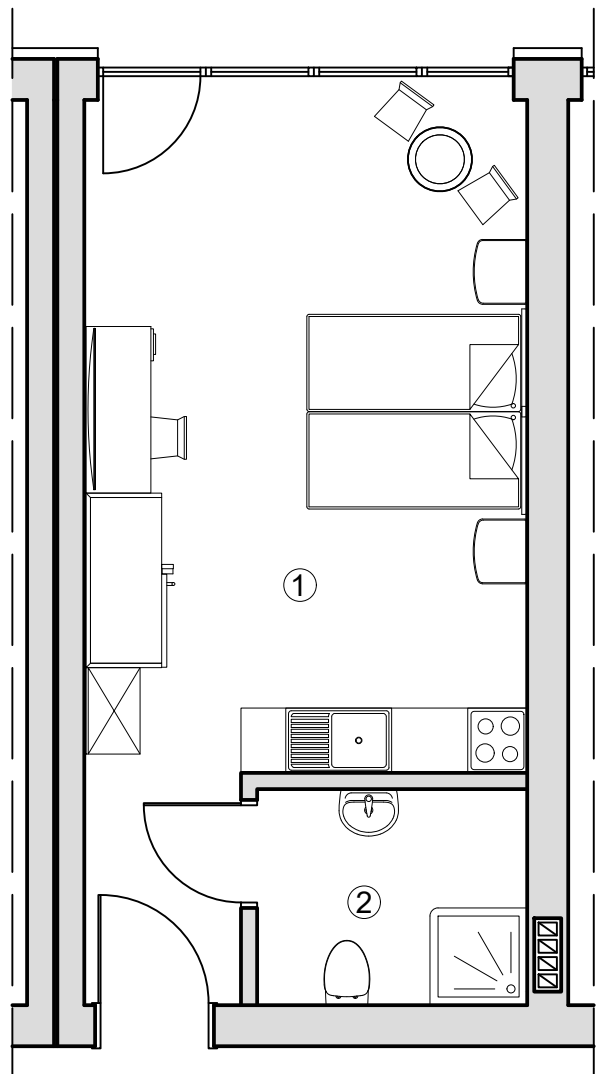
BUDYNEK HOTELU- PARTER
