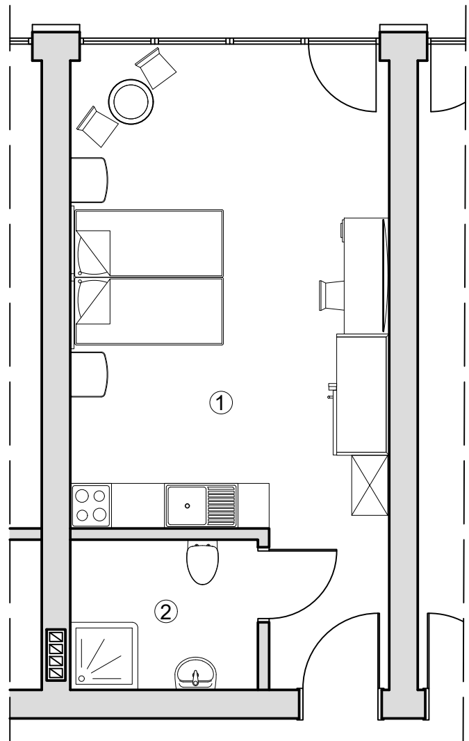
BUDYNEK HOTELU- PARTER
