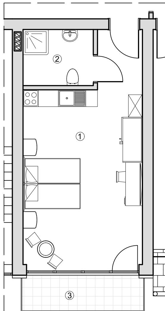
BUDYNEK HOTELU- II PIĘTRO
