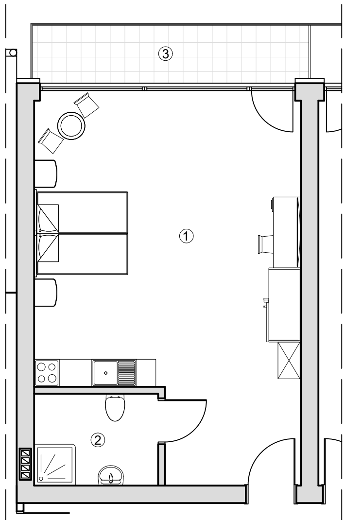
BUDYNEK HOTELU- PODDASZE
