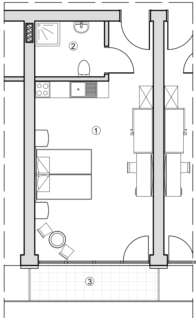
BUDYNEK HOTELU- PODDASZE
