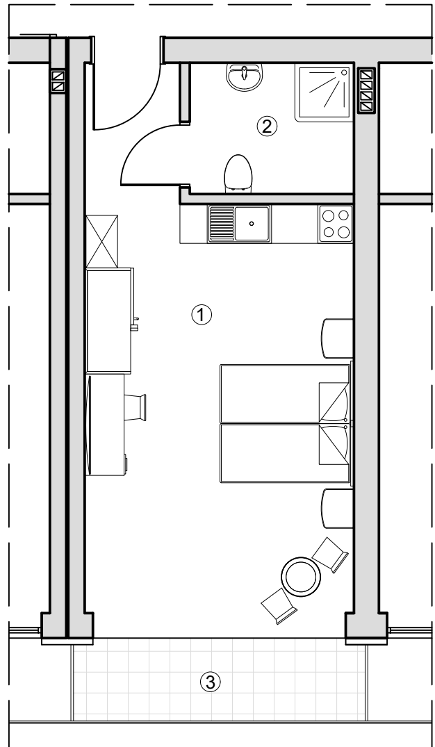
BUDYNEK HOTELU- PODDASZE
